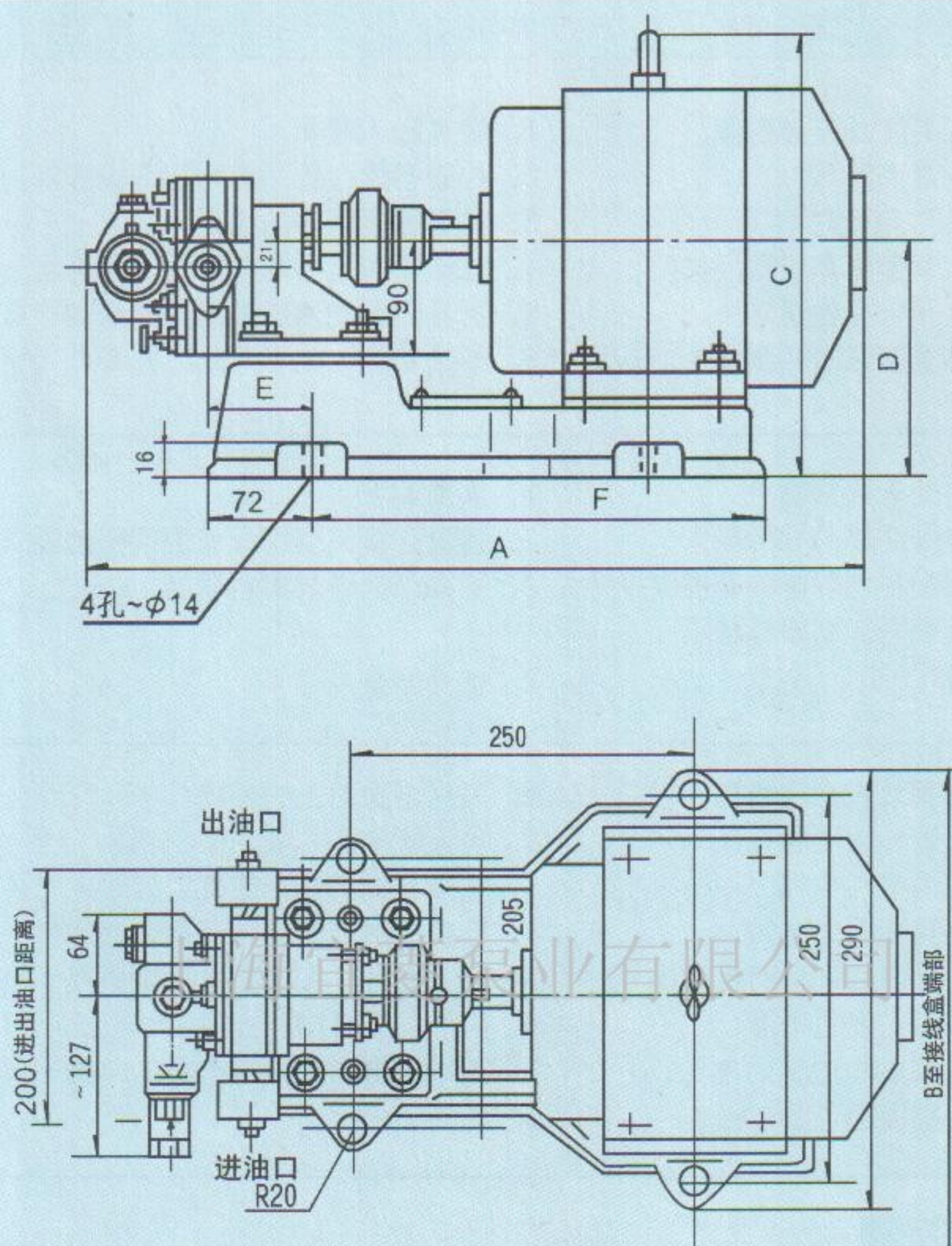
齿轮油泵外形尺寸表
