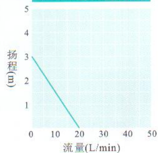
性能曲线(抽取水20℃)
