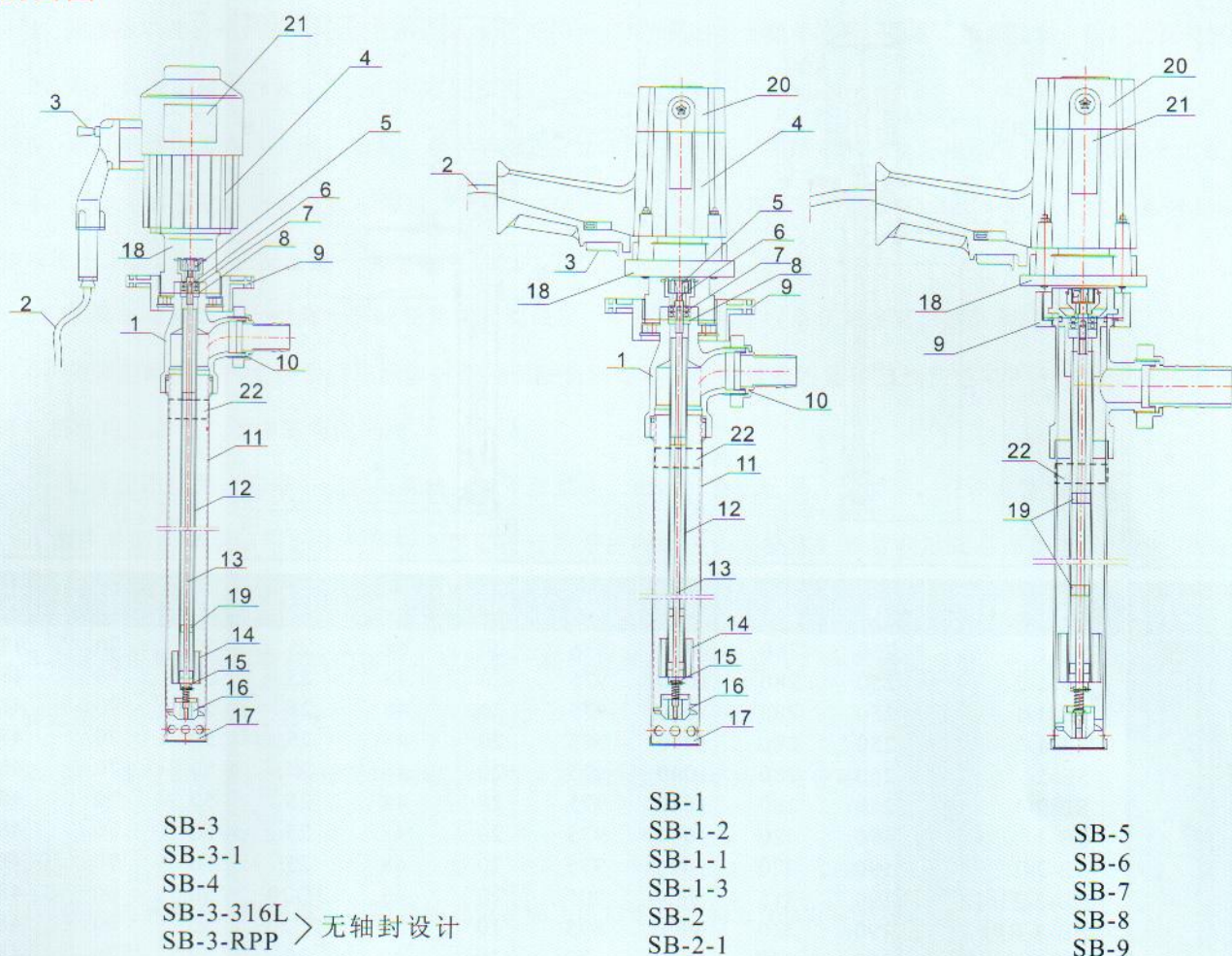
剖面图
