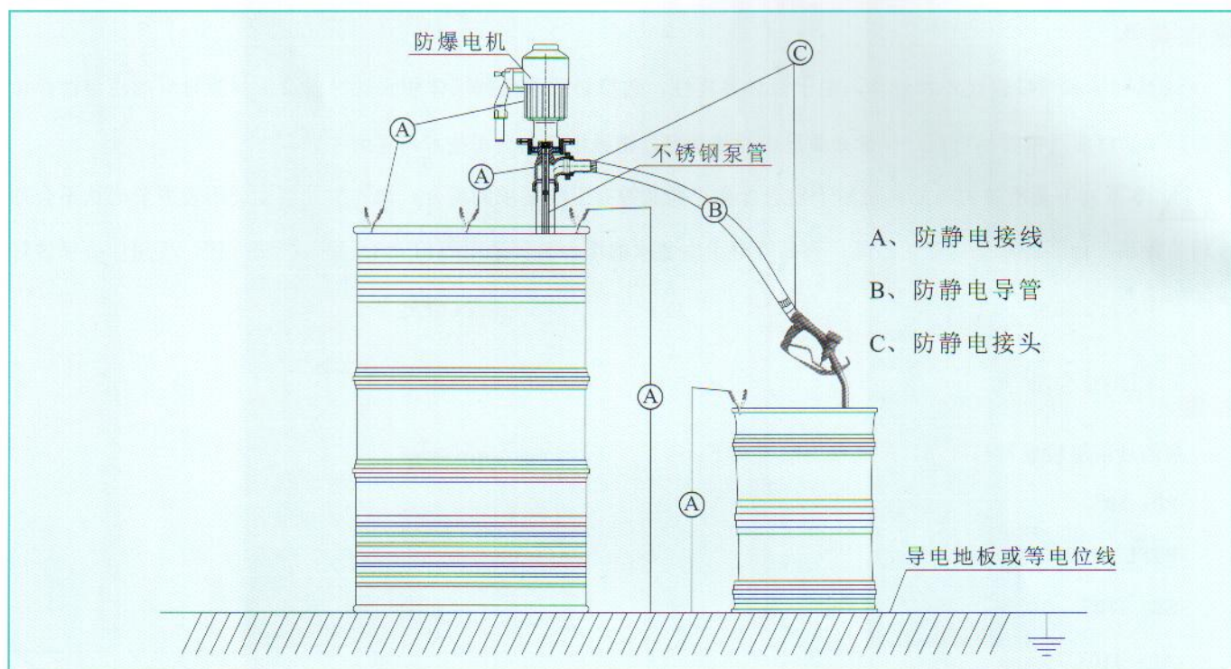
图一：防静电装置示意图
